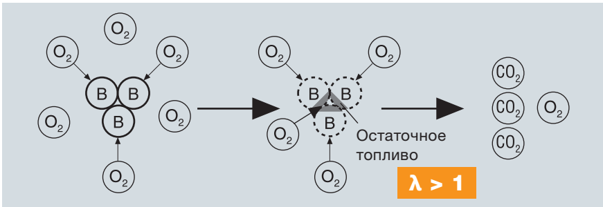
Рис. 11: Реальный процесс сгорания
