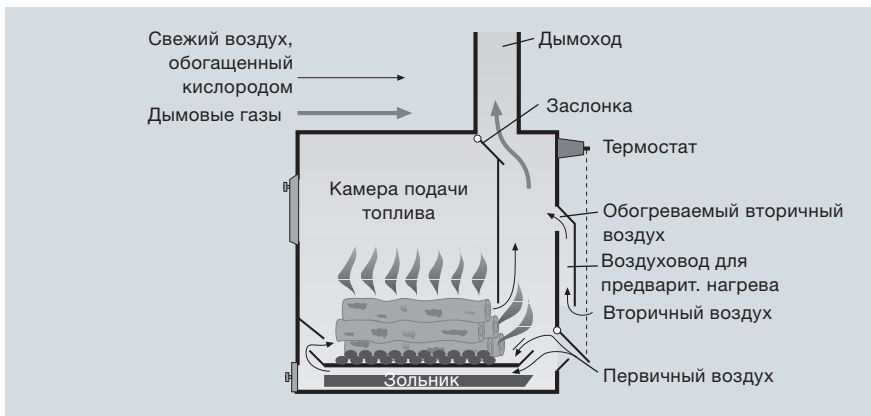
Рис. 4: Простая колосниковая печь
