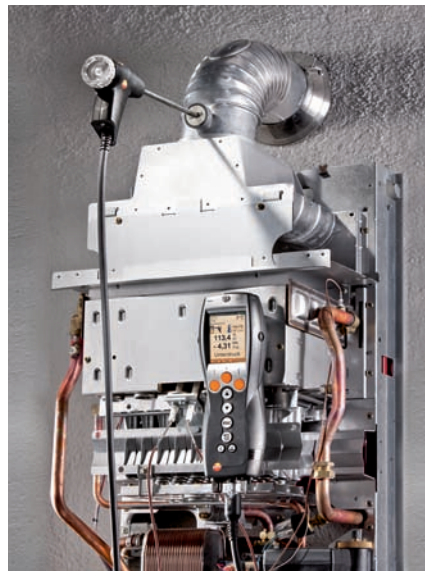
Рис. 8: Для осуществления настройки необходимо иметь анализатор дымовых газов, например, testo 330
